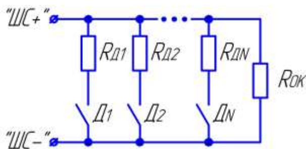
Рис.4 Схема подключения пожарных дымовых датчиков к шлейфу с типом =7 (Д1...ДN – контакты пожарных дымовых датчиков; Rок – оконечный резистор номиналом 5,6 кОм ±5%; RД1, RД2 ... RДN – добавочные резисторы номиналом 2,2 кОм ±5%. Максимальное допустимое сопротивление проводов шлейфа в данной схеме – 220 Ом; минимальное допустимое сопротивление утечки между проводами шлейфа – 7 кОм; максимальный допустимый ток утечки – 1,5 мА).
