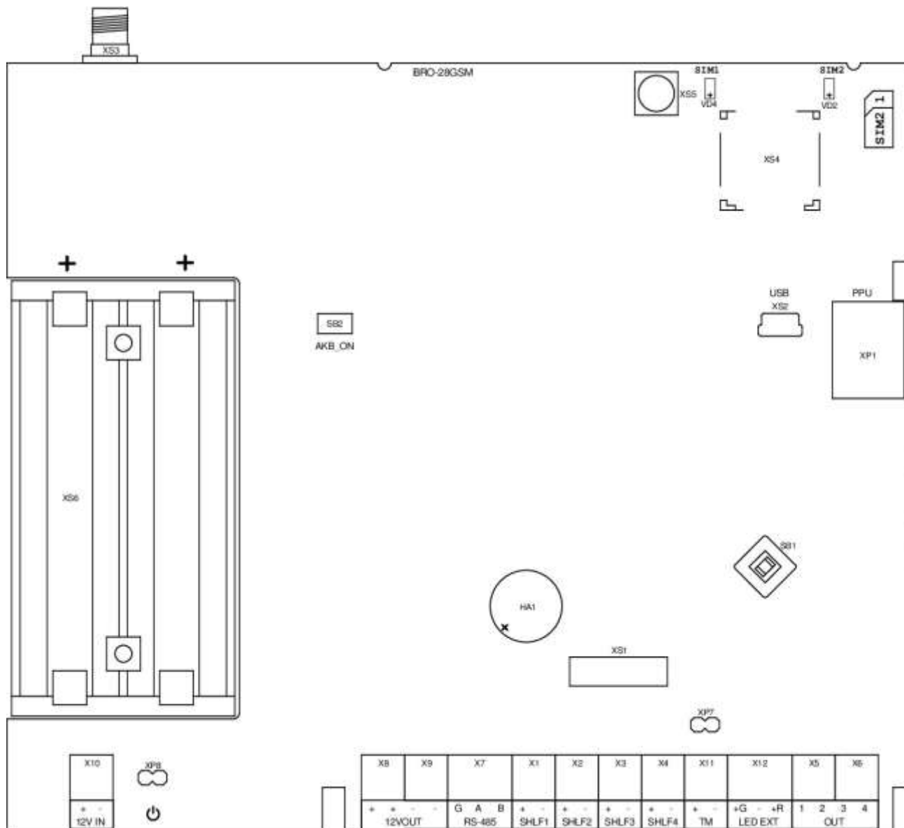
Рис.9 Внешний вид платы контроллера.
