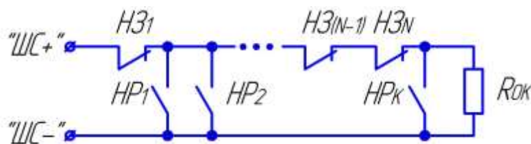
Рис.2 Схема подключения охранных датчиков (НЗ – нормально замкнутый контакт охранного датчика; НР – нормально разомкнутый контакт охранного датчика; Rок – оконечный резистор номиналом 4,7 кОм \pm 5%. Максимальное допустимое сопротивление проводов шлейфа в данной схеме – 470 Ом; минимальное допустимое сопротивление утечки между проводами шлейфа – 18 кОм; максимальный допустимый ток утечки – 0,6 мА).
