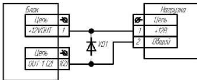
Рис.7 Подключение выходов при использовании выхода питания для внешних потребителей (Напряжение на нагрузке 11,5...12,5В, максимальный ток потребления 100мА. Диод VD1 нужен, если нагрузкой является катушка реле. Допустимое обратное напряжение диода должно быть не менее 20В)
