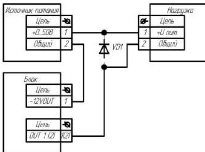
Рис.8 Подключение выходов при использовании отдельного источника питания нагрузки (Напряжение на нагрузке 0...50В, максимальный ток потребления 500мА. Диод VD1 нужен, если нагрузкой является катушка реле. Допустимое обратное напряжение диода должно превышать напряжение источника питания)
