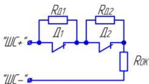
Рис.5 Схема подключения пожарных тепловых датчиков к шлейфу с типом =15 (Д1, Д2 – контакты пожарных тепловых датчиков; Rок – оконечный резистор номиналом 4,3 кОм ±5%; RД1, RД2 – добавочные резисторы номиналом 6,8 кОм ±5%. Максимальное допустимое сопротивление проводов шлейфа в данной схеме – 220 Ом; минимальное допустимое сопротивление утечки между проводами шлейфа – 50 кОм; максимальный допустимый ток утечки – 0,21 мА).
